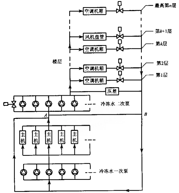
图 1 大厦冷冻水管网示意图
