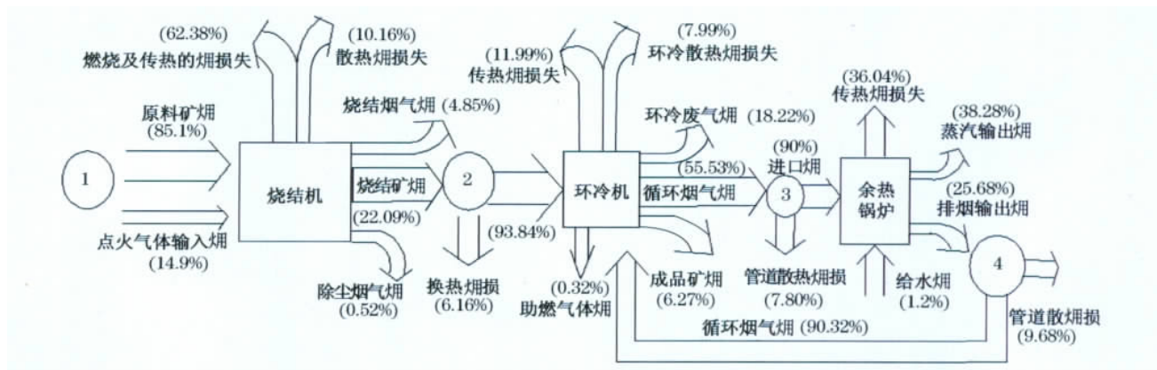
图 3 烧结系统烟流分布图
