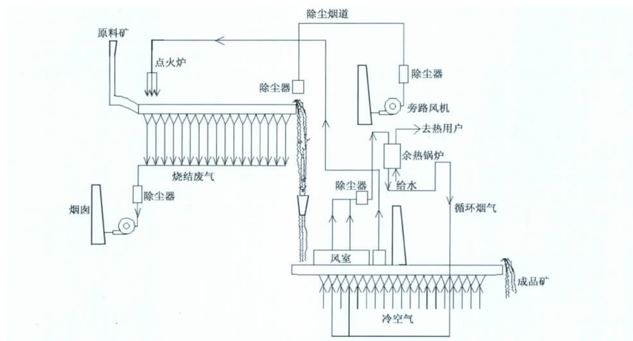
图 2 某厂烧结余热回收系统流程图
